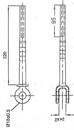
(2) STEEL DEAD END
